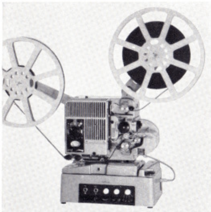
Tonfilm-Projektor »2000«
