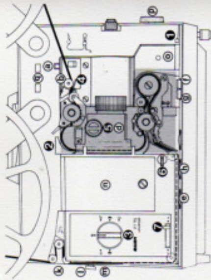
Abgebildet ist der Projektor P 7 TS universal
